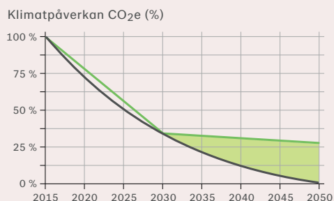
Figur 2. Potential för att minska klimatpåverkan från odlingen, beräknat per ton höstvet, samt gap mot Parisavtalet. ● Potential för CO 2 e minskning ● Minskningstakt för klimatpåverkan, enligt Parisavtalet ■ Innovationsgap
